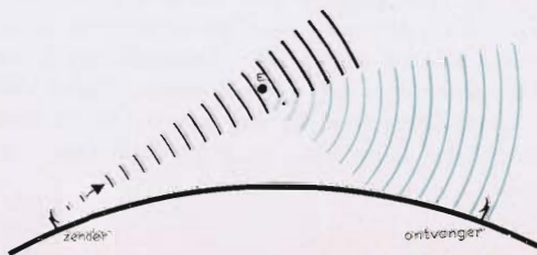
Fig. 18. Kunstmanen worden gebruikt voor het overbrengen van signalen over grote afstand.
