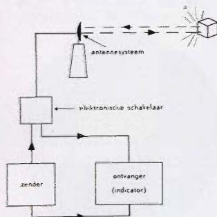
Fig. 11. Schema van een radarinstallatie
