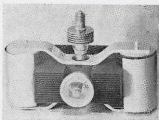
Fig. 8. Een magnetron
