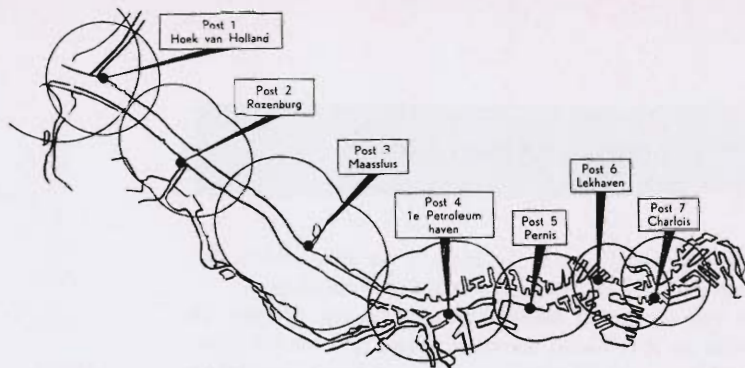
Fig. 17. De havenradar-keten met zeven stations langs de Nieuwe Waterweg
